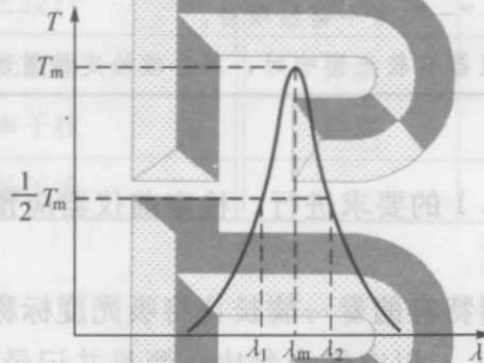
图 1 波长-透射比特性曲线
